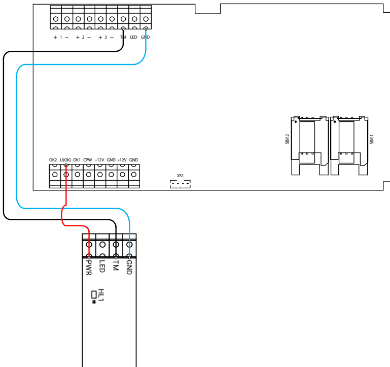
Рисунок 13. Схема подключения считывателя «MIF2-1»
