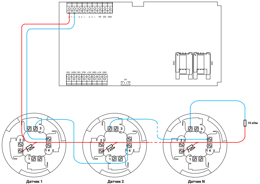
Рисунок 10. Схема подключения пожарных шлейфов с контролем обрыва
