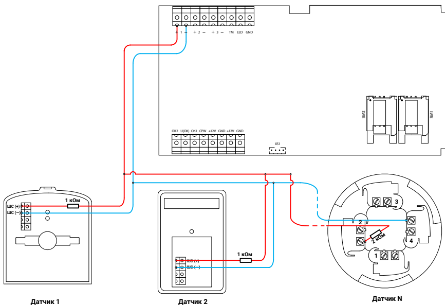
Рисунок 11. Схема подключения ручных пожарных извещателей
